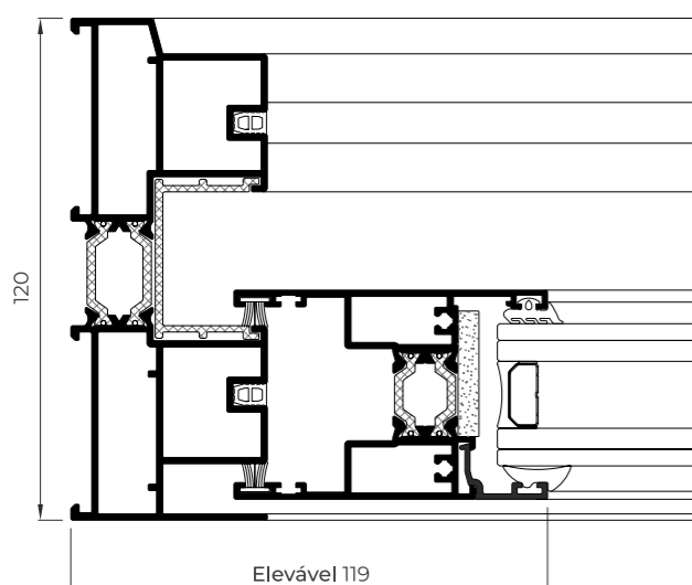
Seção lateral
