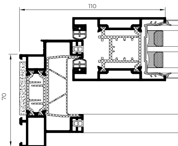
Seção lateral
